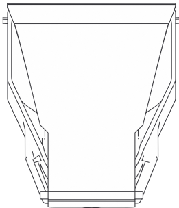
REAR · W 43 MM · H 47 MM
